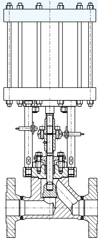
Absperrventil mit pneum. Antrieb
