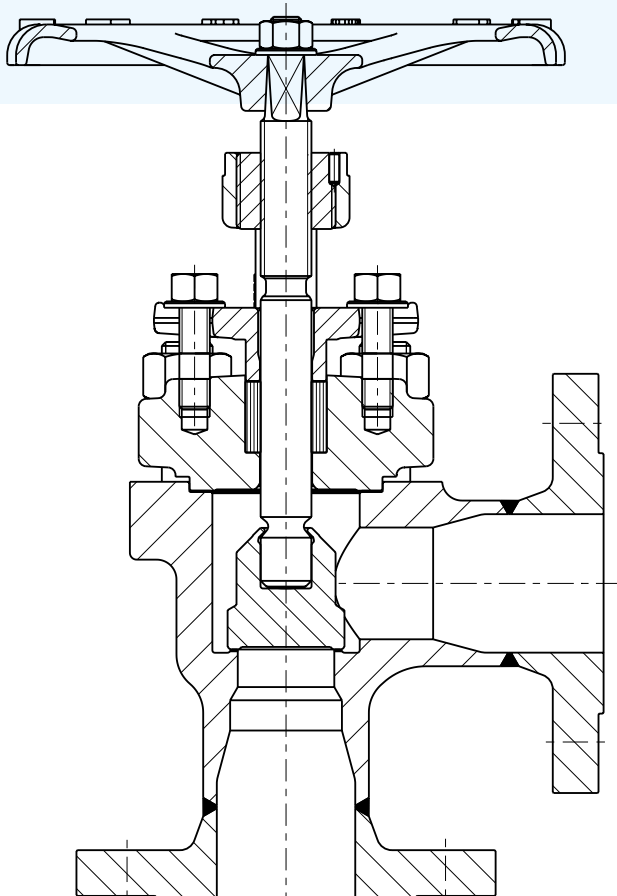
Eckventil 202 AE
