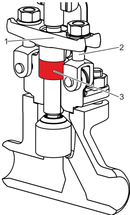
Abb. 9: Stopfbuchspackung
