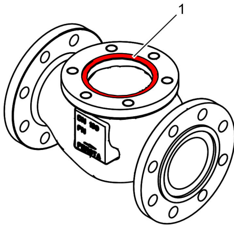
Abb. 29: Deckeldichtung
