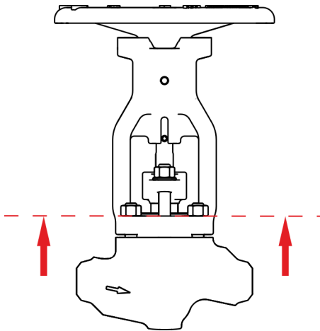
Abb. 20: Oberkante der Isolierung
