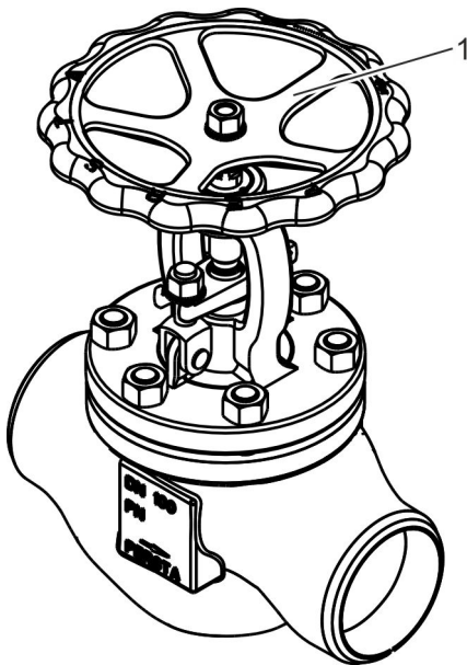
Abb. 12: Manueller Antrieb
