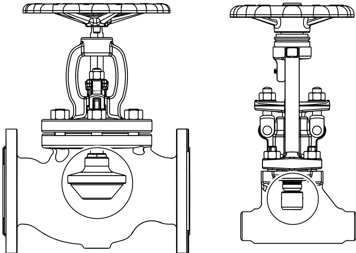
Abb. 1: Absperrventile mit unterschiedlichen Absperrorganen
