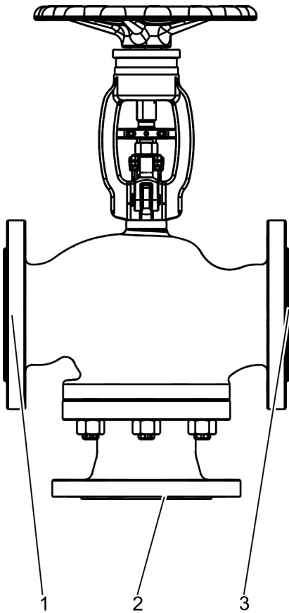
Abb. 17: Drei Flanschverbindungen
