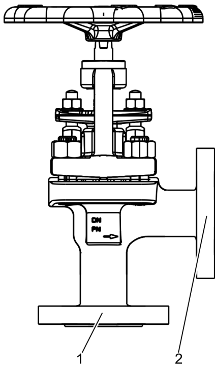
Abb. 16: Eckventil
