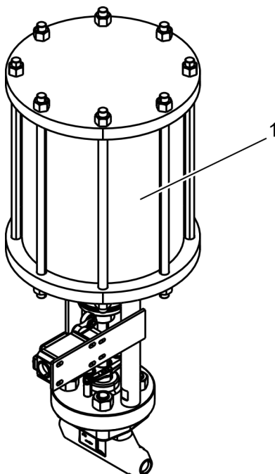
Abb. 14: Pneumatischer Antrieb
