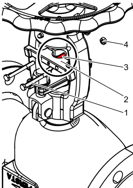
Abb. 41: Schalterklaue montieren
