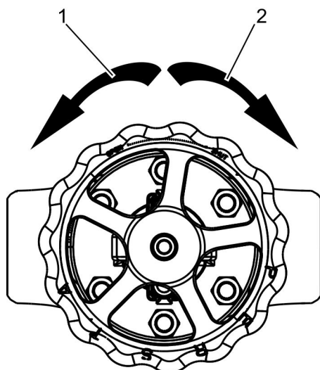
Abb. 23: Manueller Antrieb: Handrad im Notfall betätigen
