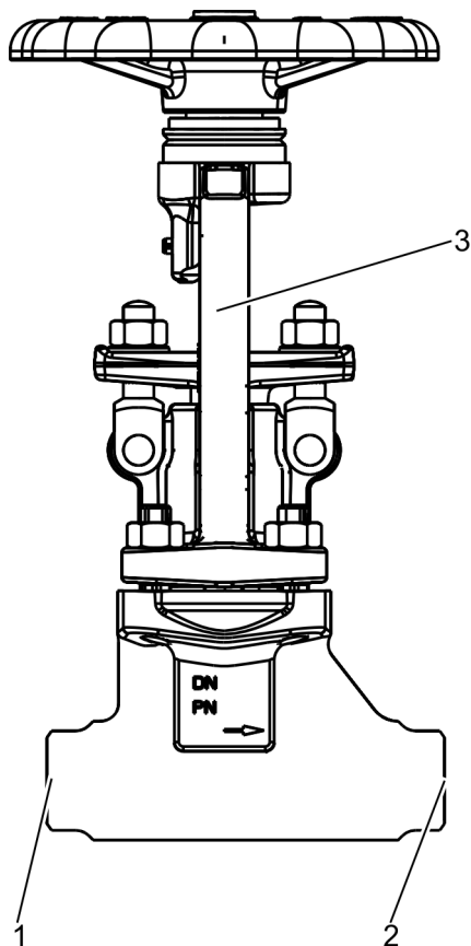
Abb. 15: Durchgangsform
