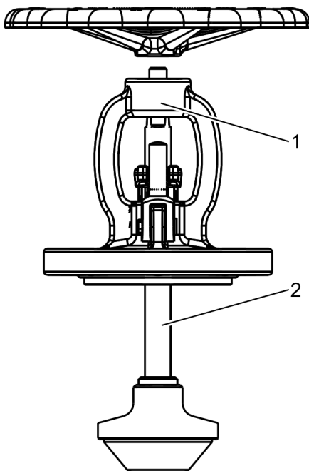
Abb. 30: Spindel herausdrehen
