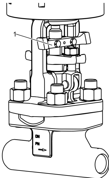
Abb. 5: Mechanische Stellungsanzeige
