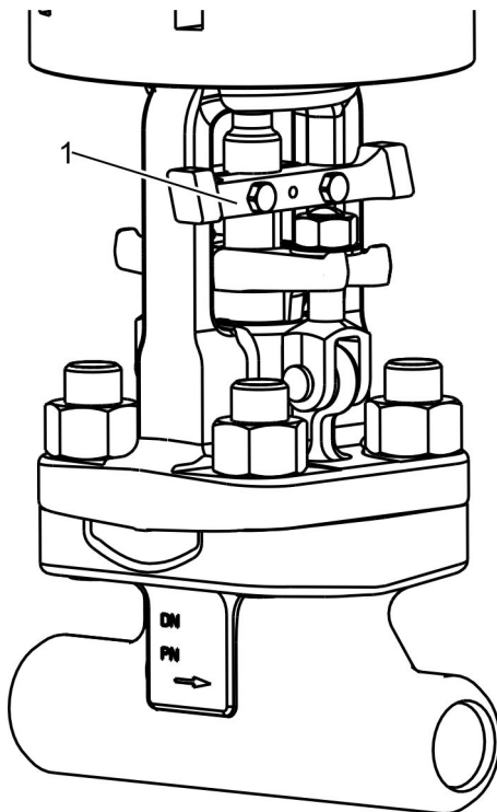
Abb. 19: Mechanische Stellungsanzeige
