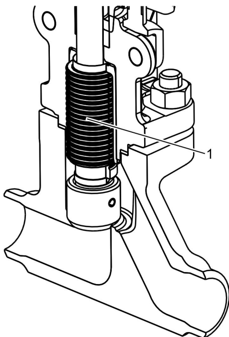
Abb. 10: Faltenbalg
