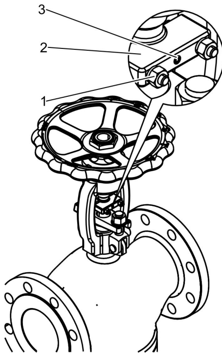
Abb. 39: Verschraubungen lösen
