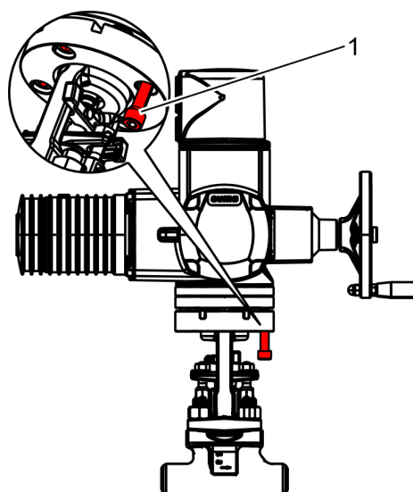
Abb. 38: Elektrischen Antrieb befestigen
