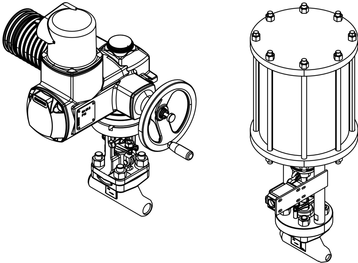
Abb. 2: Optionale Antriebe
