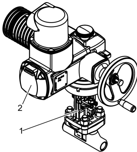
Abb. 13: Elektrischer Antrieb
