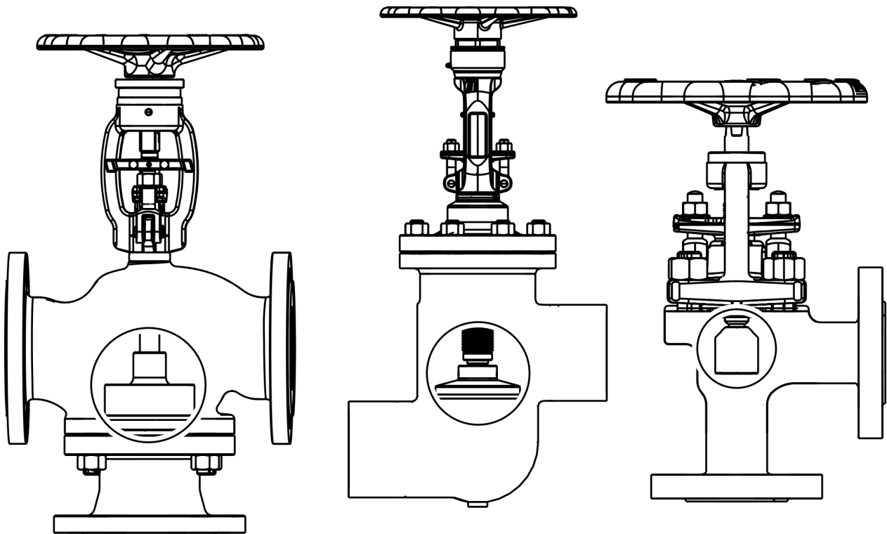
Abb. 3: Unterschiedliche Gehäuseformen
