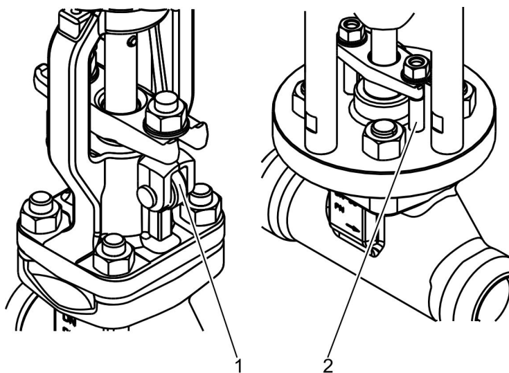
Abb. 11: Stopfbuchsschrauben
