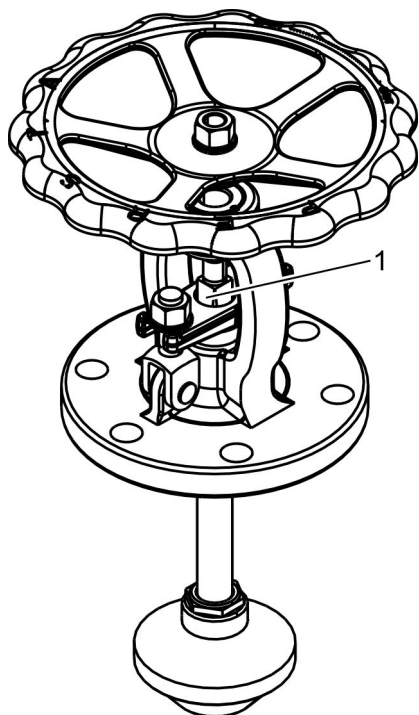
Abb. 33: Spindel eindrehen
